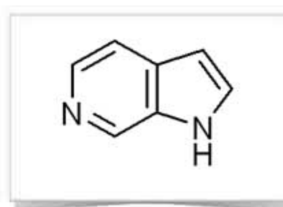
6-Azaindole
