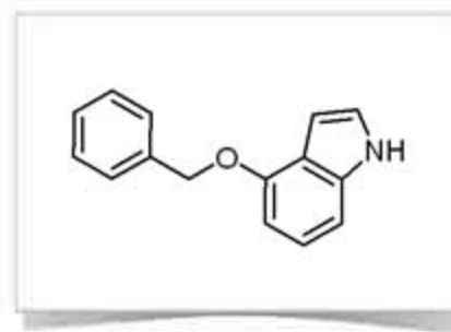
4-Benzyloxyindole
