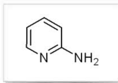
2-Aminopyridine
