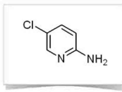
2-Amino-5-chloropyridine
