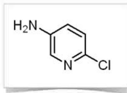
5-Amino-2-chloropyridine
