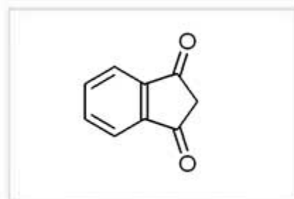
1,3 - Indanedione
