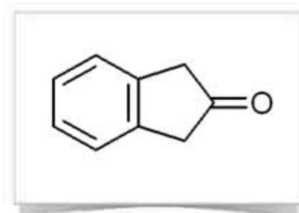
2-Indanone
