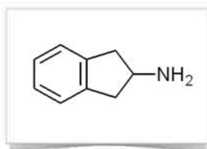
2-aminoindane
