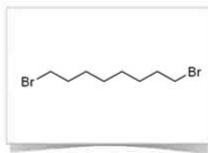
1,8-dibromooctane
