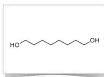
1,8-Octanediol
